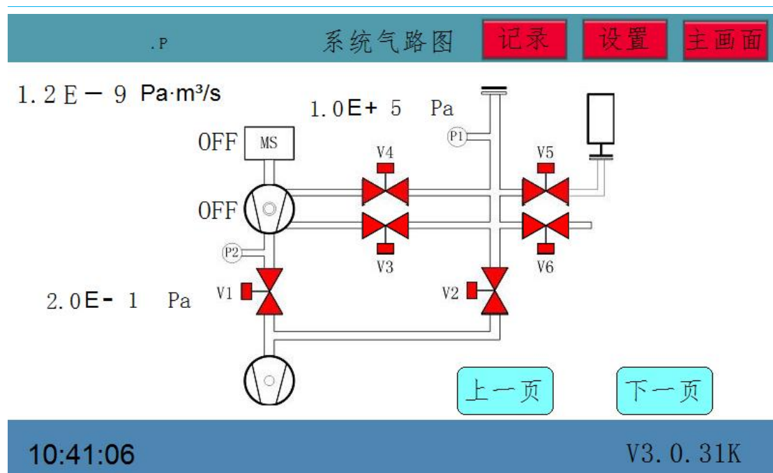
图 27 系统气路图
