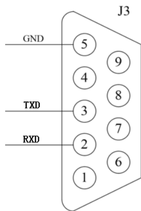
RS232 接口
