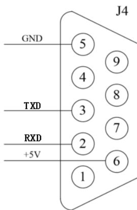
遥控器接口
