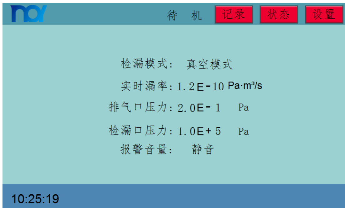
图 11 待机界面
