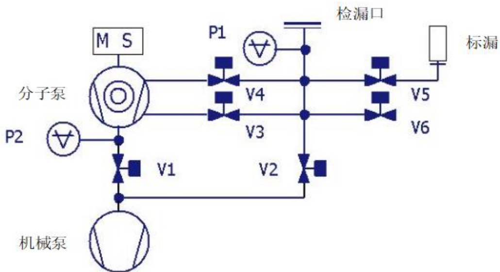
图6 气路图
