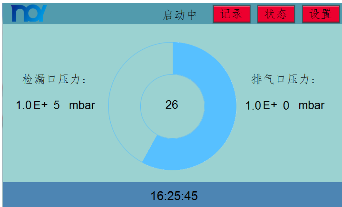
图 10 启动界面
