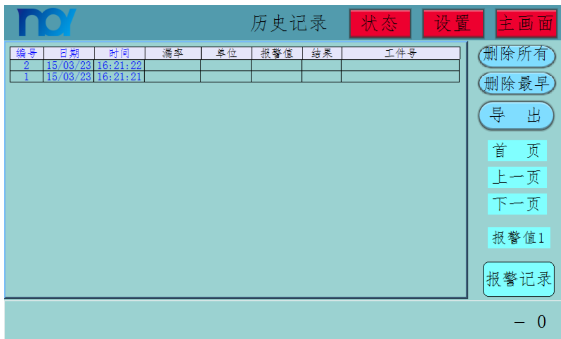
图 22 记录界面
