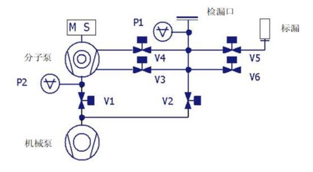
图 6 气路图
