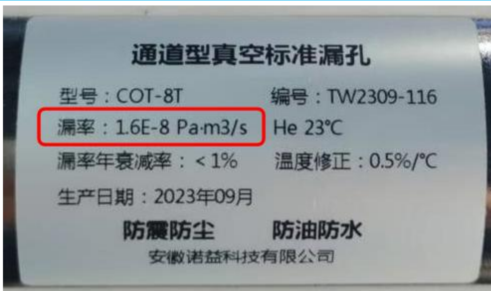
图 42 标漏铭牌
