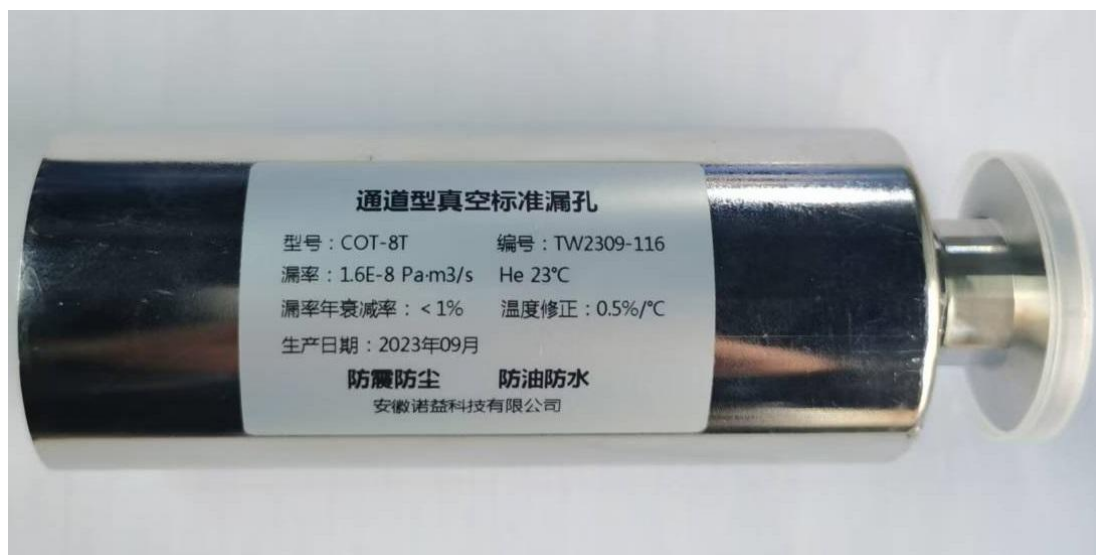
图 35 标准漏孔
