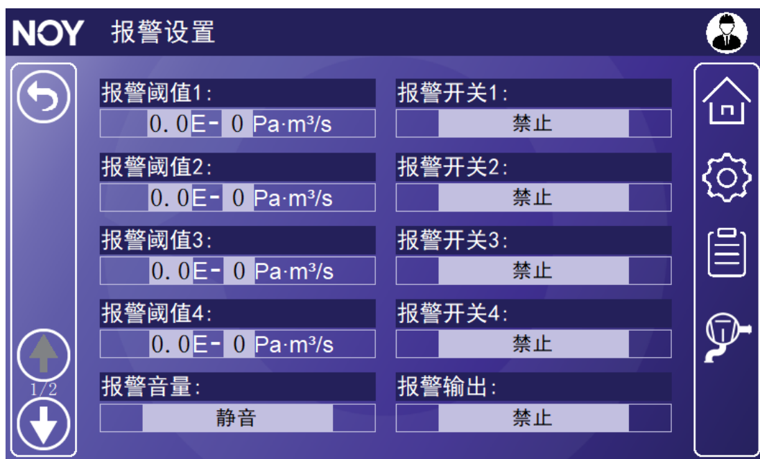
图 13 报警设置界面 1
