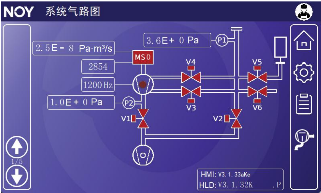
图 33 系统气路图
