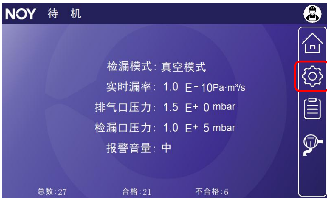
图 36 待机界面
