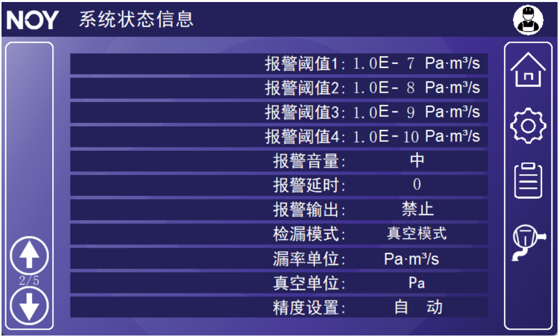
图 30 状态界面 1
