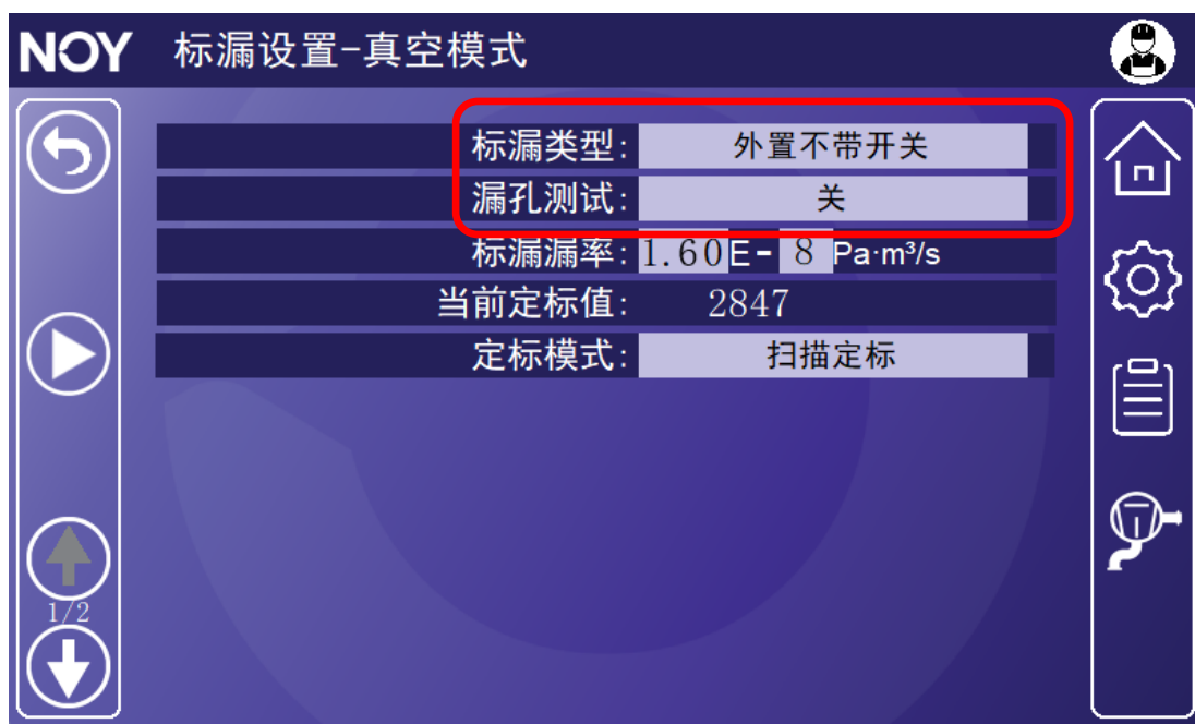
图 40 标漏类型设置
