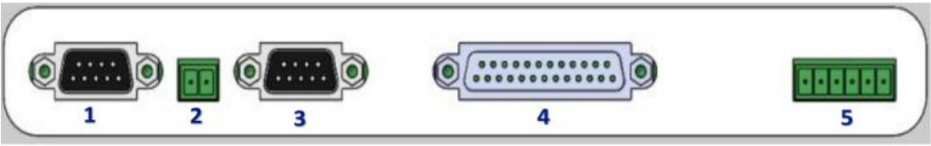
图 7 信号接口图
